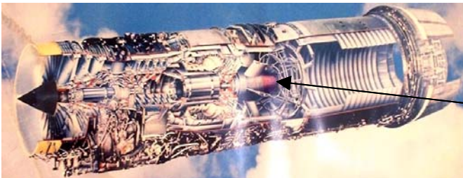
MOTEUR M53 MIRAGE
